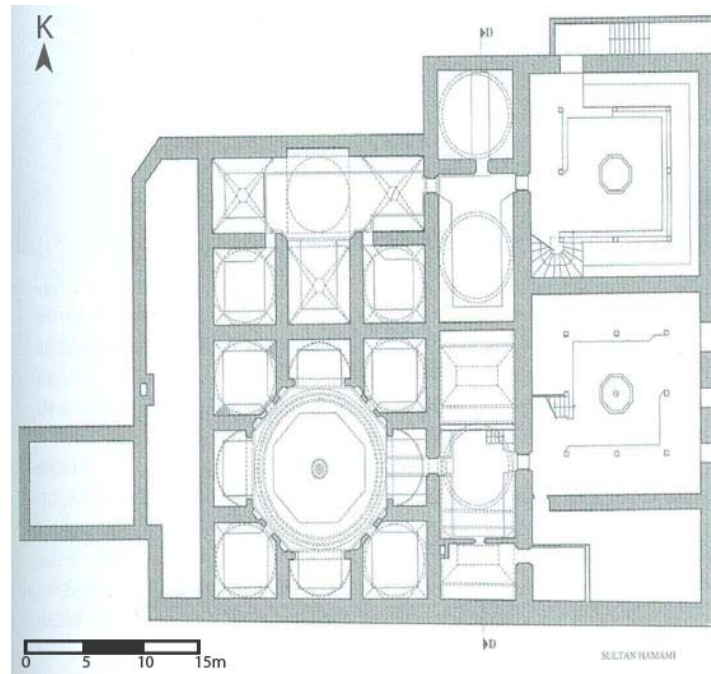
Krş. Planı 5.4: Tokat Sultan Hamamı (O. Eravşar'dan)
