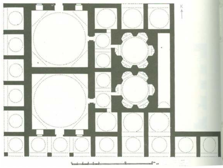
Krş. Planı 5.31: Lüleburgaz Sokullu Mehmet Paşa Hamamı (Y. Önge'den)
