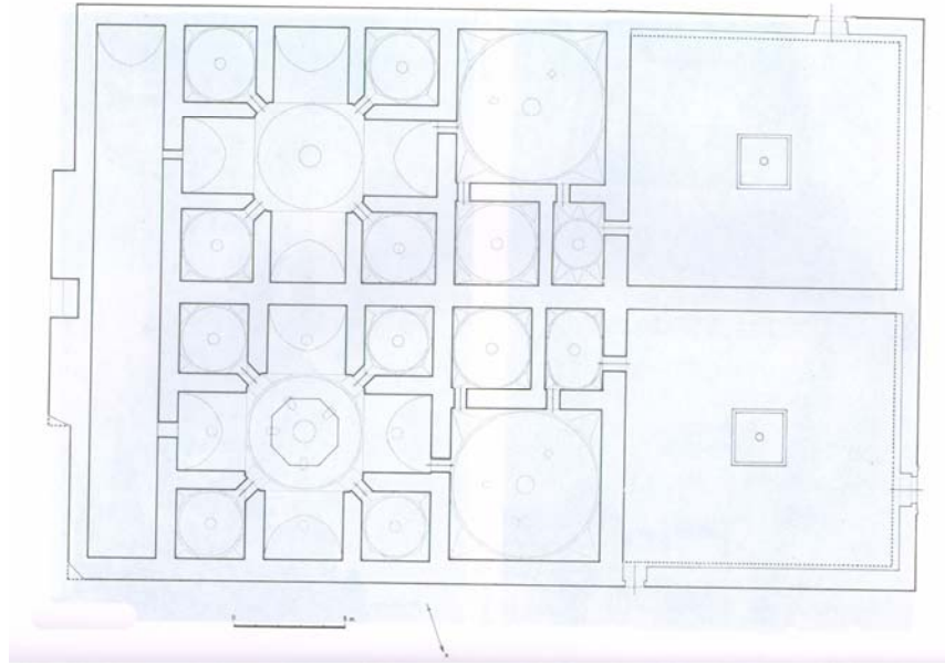
Krş. Planı 5.3: Konya Sahip Ata Hamamı (Y. Önge'den)
