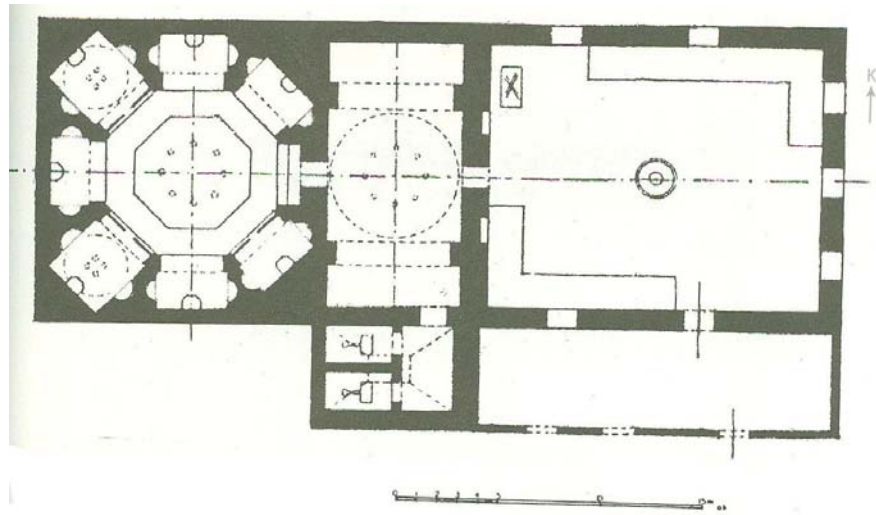
Krş. Planı 5.32: İzmit Hüsrev Kethüda Hamamı (Y. Önge'den)
