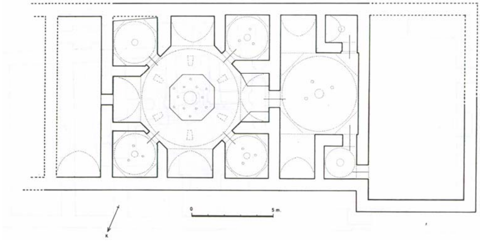
Krş. Planı 5.7: Ermenek Karamanoğlu Mahmud Bey Hamamı (Y. Önge'den)
