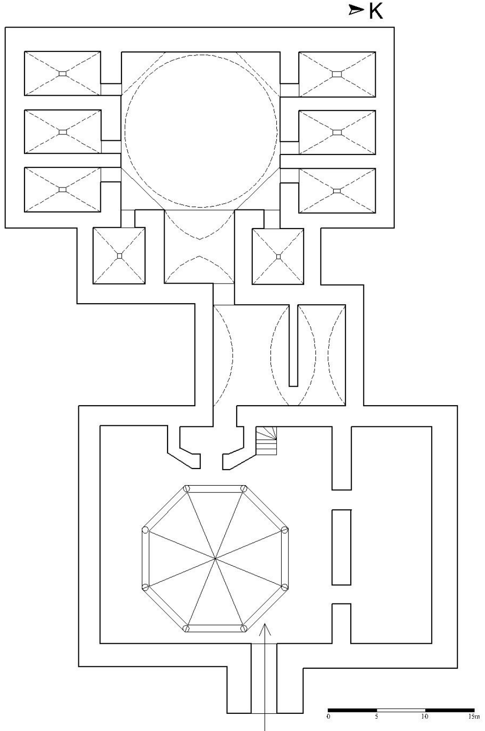
Plan 4.12: Erzurum Hamamı (Pastırmacı-Fuadiye Hamamı) (R.H.Ünal'dan düzeltilerek)
