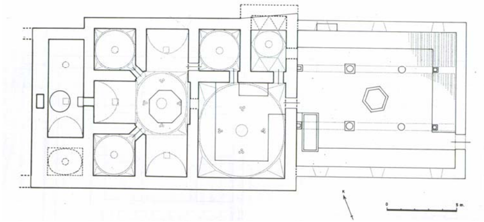
Krş. Planı 5.18: Sivrihisar Seydiler Hamamı (Y. Önge'den)
