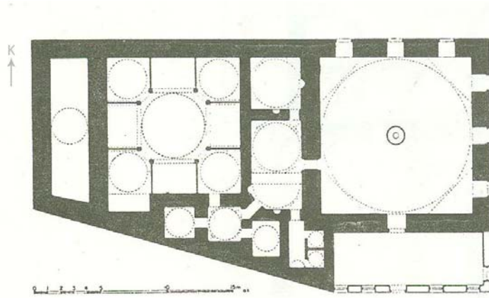
Krş. Planı 5.12: İstanbul Süleymaniye Külliyesi Hamamı (O. Aslanapa'dan)
