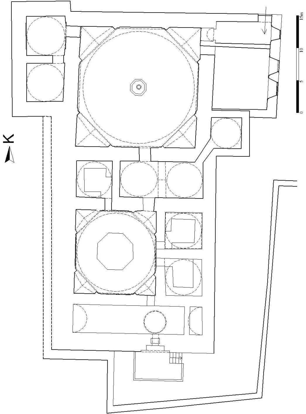
Plan 4.18: Erzurum Saray Hamamı (V.G.M.'den)
