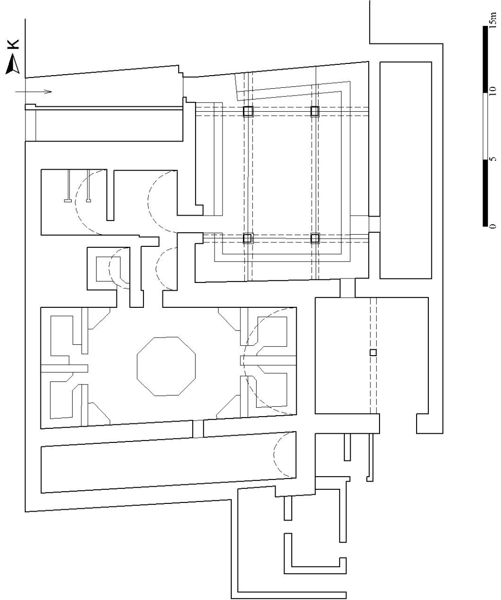
Plan 4.16: Erzurum Tahta Hamamı (V.G.M.'den)
