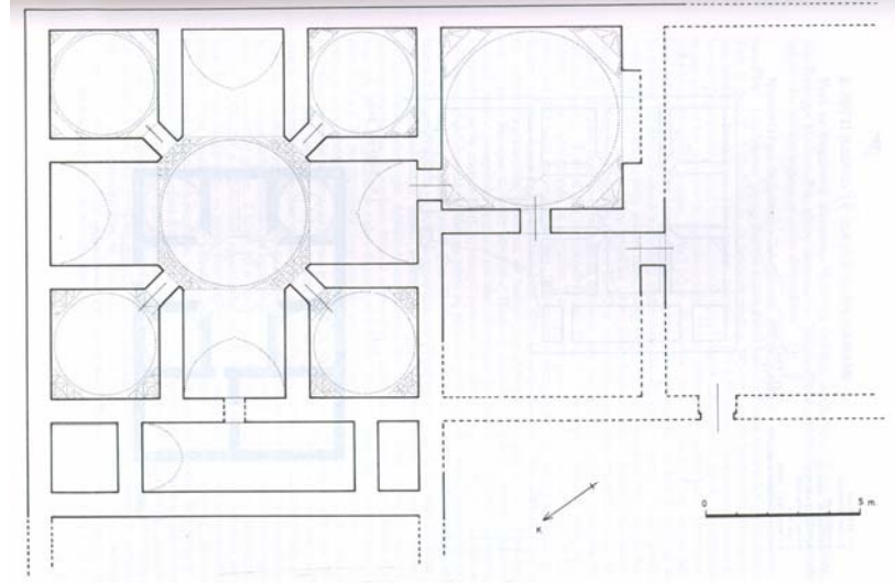
Krş. Planı 5.1: Ani Menuçerh Hamamı (K. Balkan'dan)
