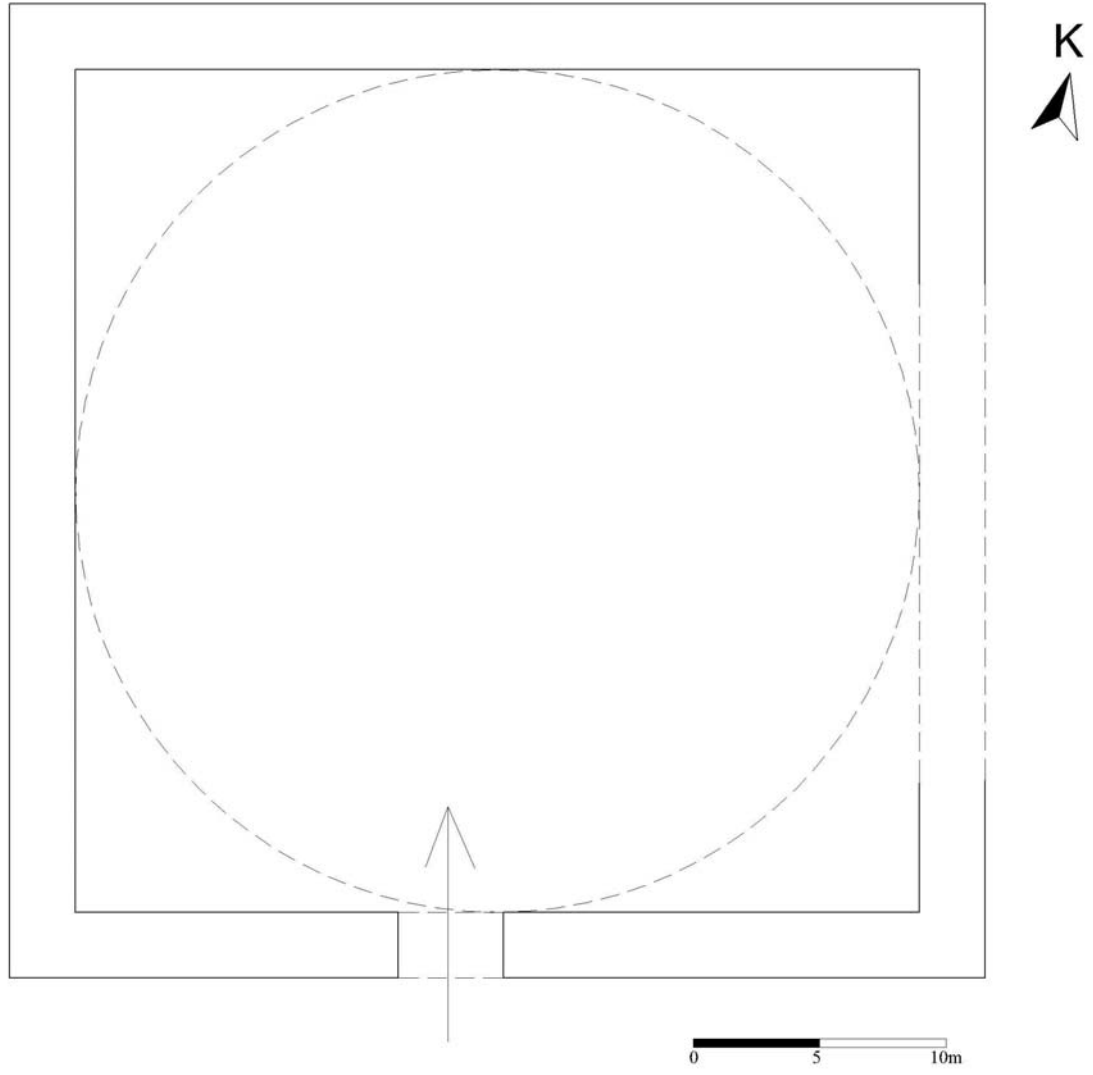
Plan 4.22: Oltu Arslan Paşa Hamamı
