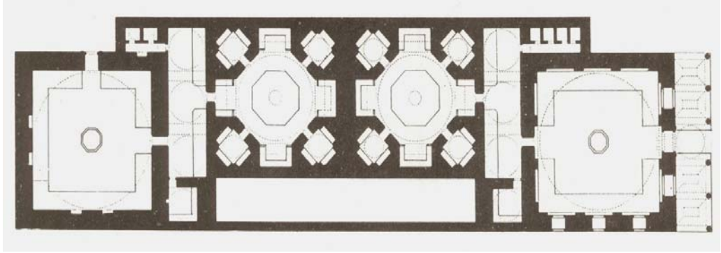
Plan 2.5: Çift Fonksiyonlu Hamam (İstanbul Haseki Hürrem Sultan Hamamı (O. Aslanapa'dan))
