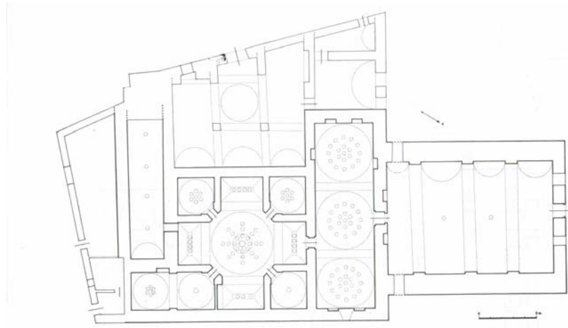
Krş. Planı 5.8: Kayseri Selâhaddin Hamamı Hamamı (Y. Önge'den)
