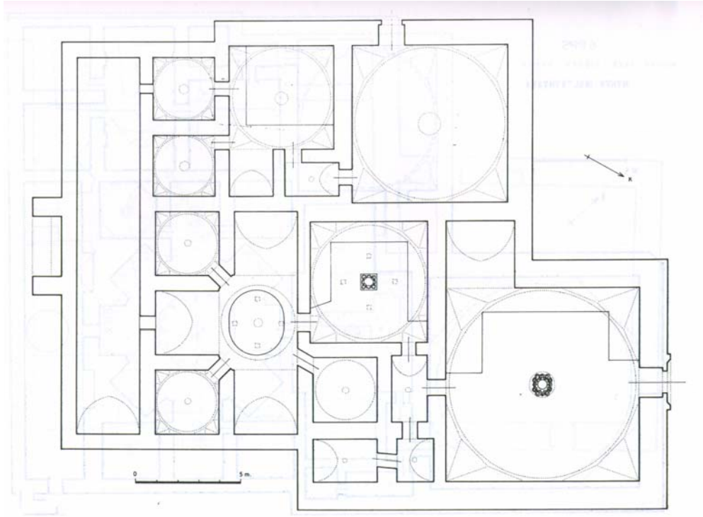
Krş. Planı 5.19: Karaman Sekizçeşme Hamamı (Y. Önge'den)
