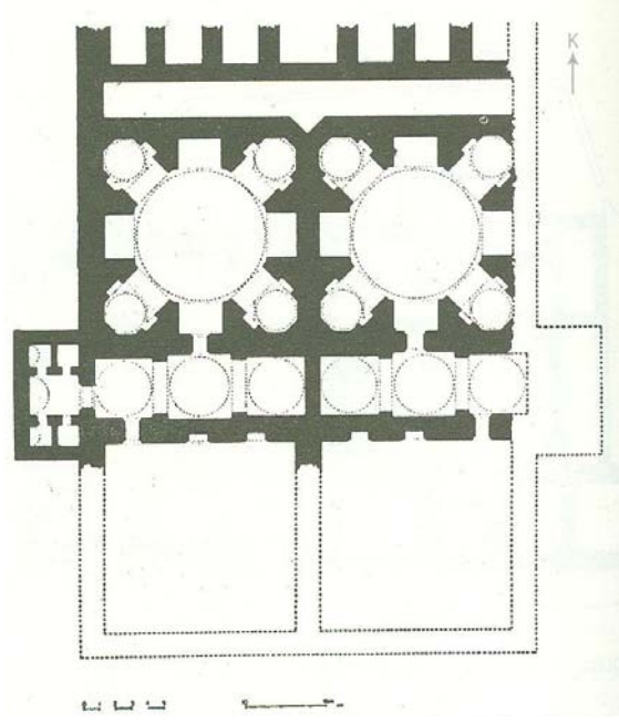
Krş. Planı 5.27: Üsküdar Atik Valide Hamamı (Y. Önge'den)
