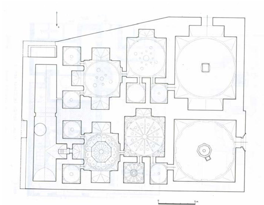
Krş. Planı 5.20: Konya Meram Hasbeyoğlu Hamamı (Y. Önge'den)
