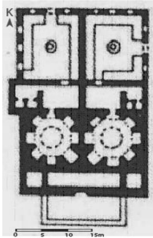
Krş. Planı 5.28: İzmit Pertev Paşa Hamamı (O. Aslanapa'dan)
