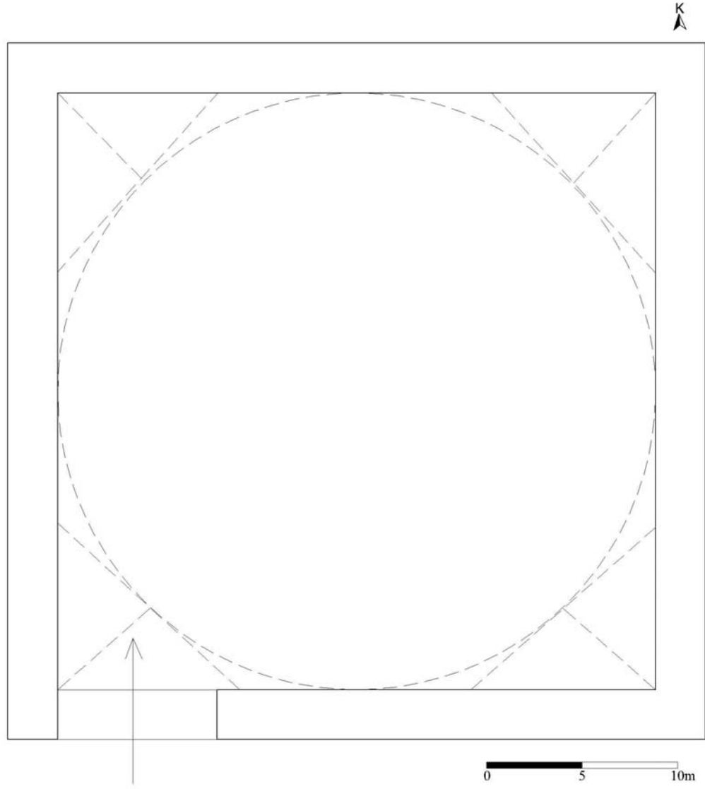
Plan 4.21: Oltu Ünlükaya Köyü Hamamı
