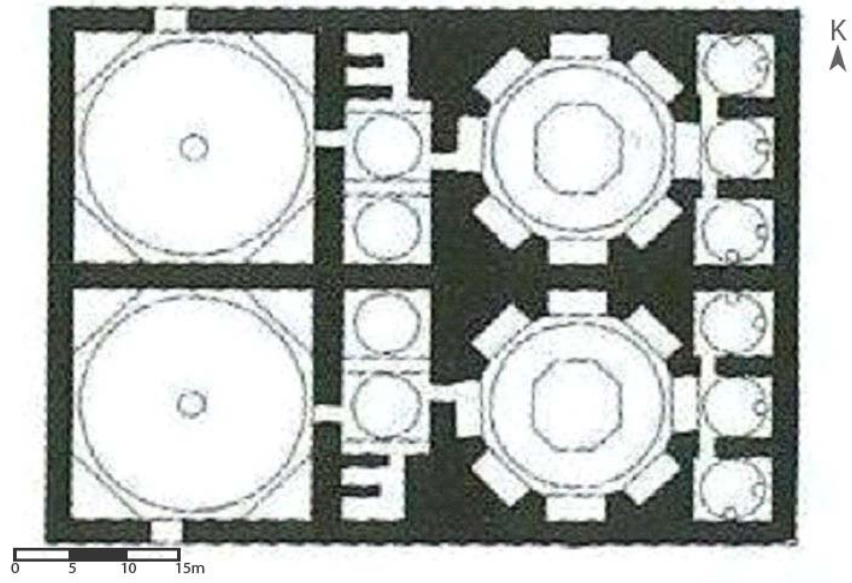
Krş. Planı 5.25: Manisa Hafsa Sultan Hamamı (D. Kuban'dan)
