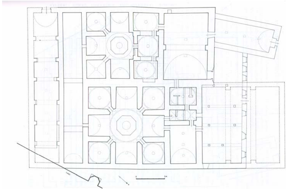
Krş. Planı 5.2: Kayseri Hunad Hamamı (Mahperi Sultan) (Y. Önge'den)
