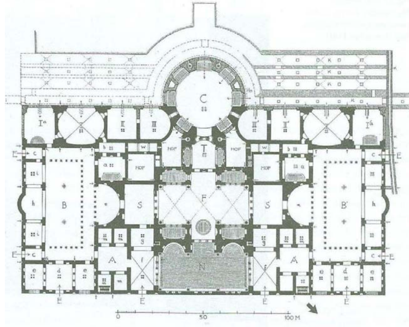
Plan 2.3: Caracalla Hamamları, Roma (F. Yegül'den)
