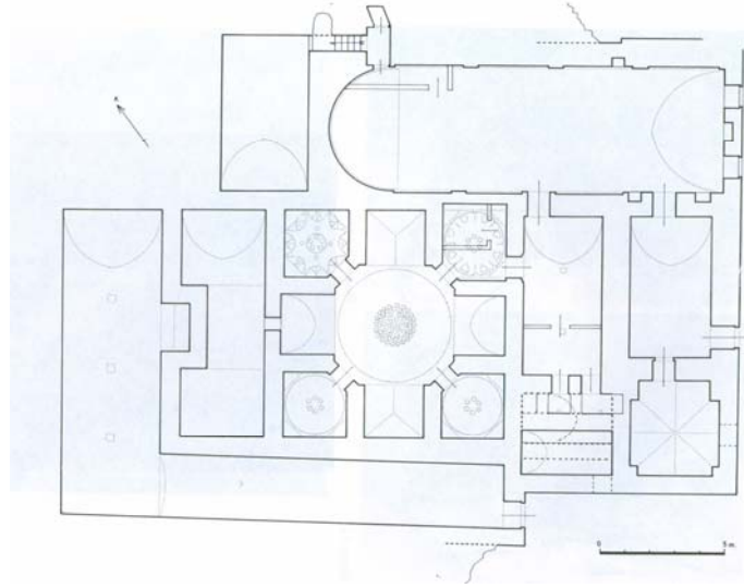
Krş. Planı 5.15: Mardin Radviyye Hamamı (Y. Önge'den)
