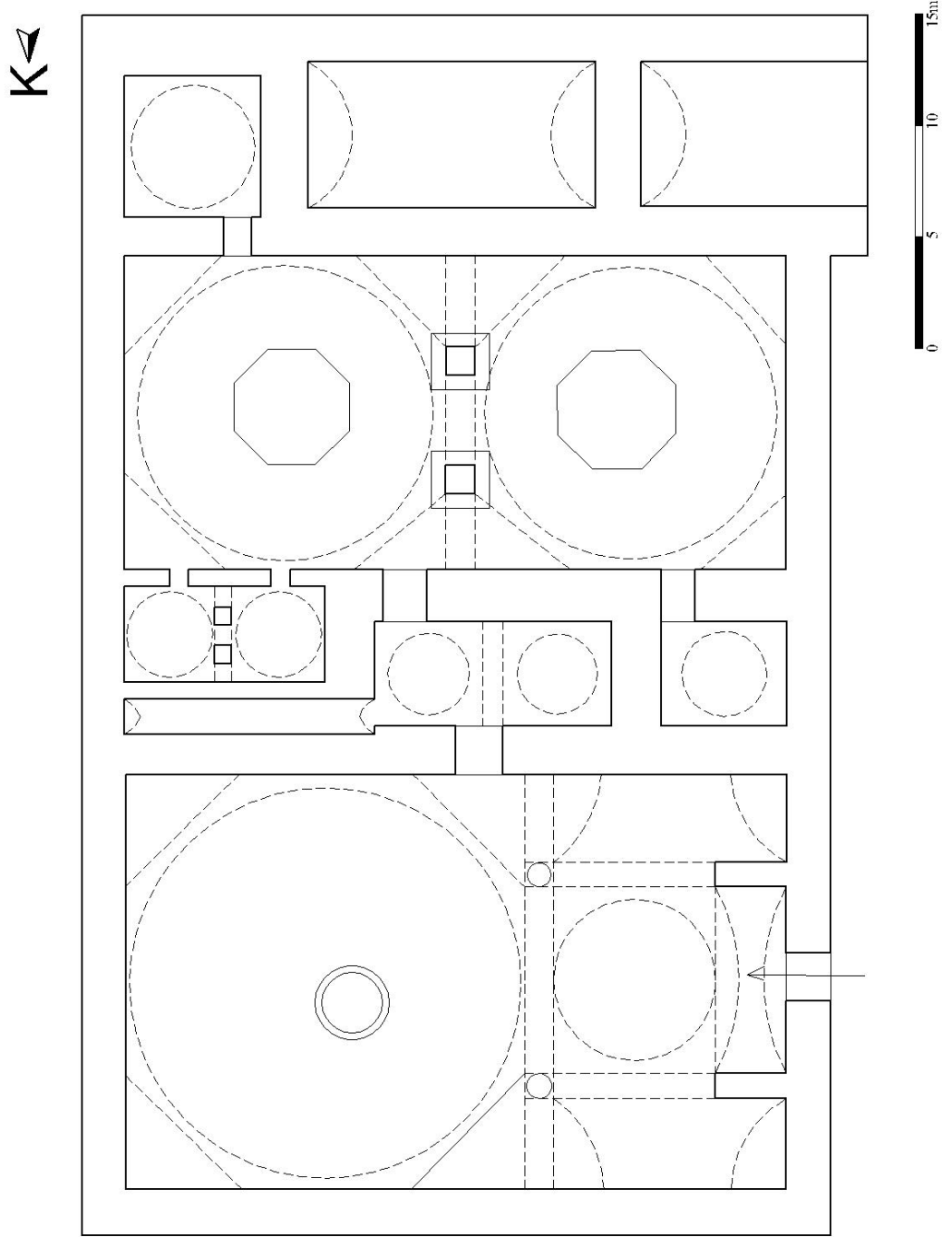
Plan 4.14: Erzurum Çifte Göbek Hamamı (R.H.Ünal'dan düzeltilerek)
