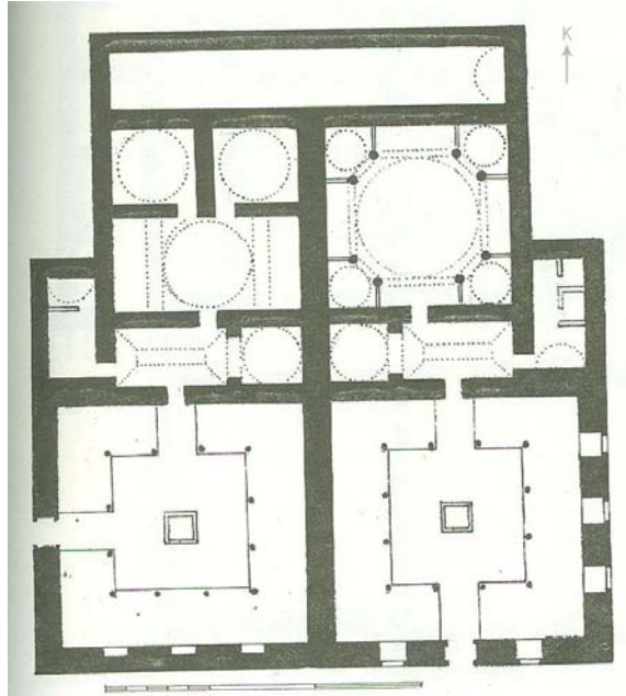
Krş. Planı 5.14: Azapkapı Sokullu Mehmet Paşa Külliyesi Hamamı (Y. Önge'den)
