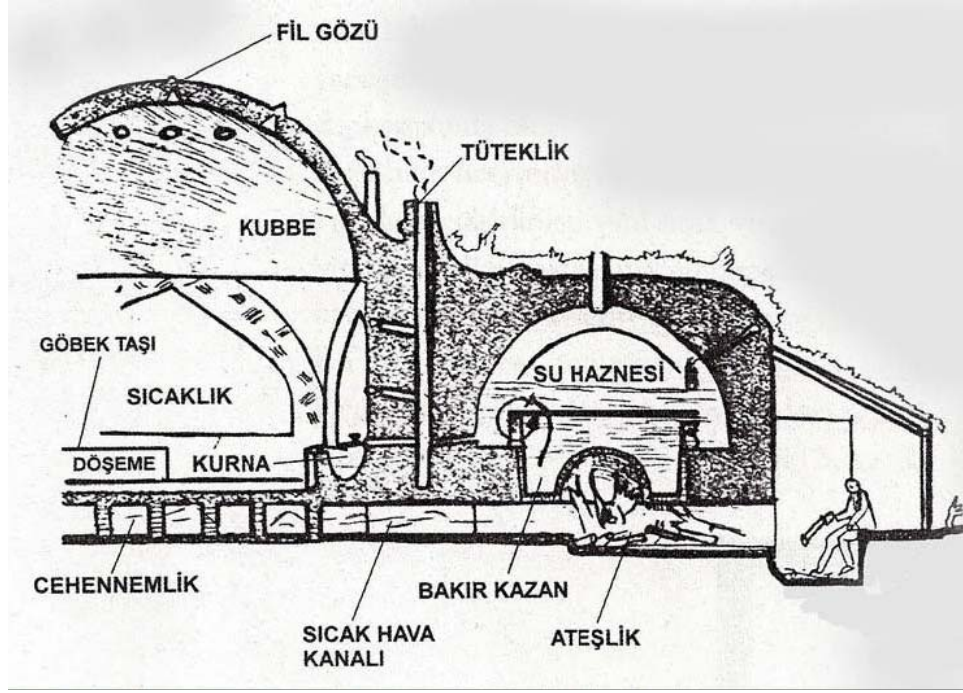
Çizim 2.7: Külhan (K. Aru'dan)
