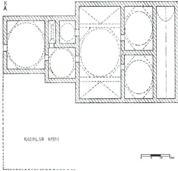
Krş. Planı 5.35: Manisa Dilşikar Hamamı (H. Acun'dan)
