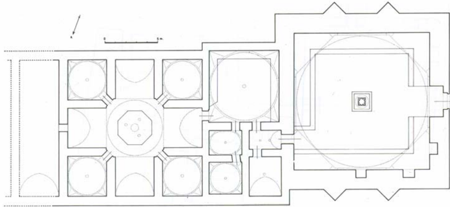
Krş. Planı 5.6: Konya Karaman Emir Süleyman Hamamı (Y. Önge'den)
