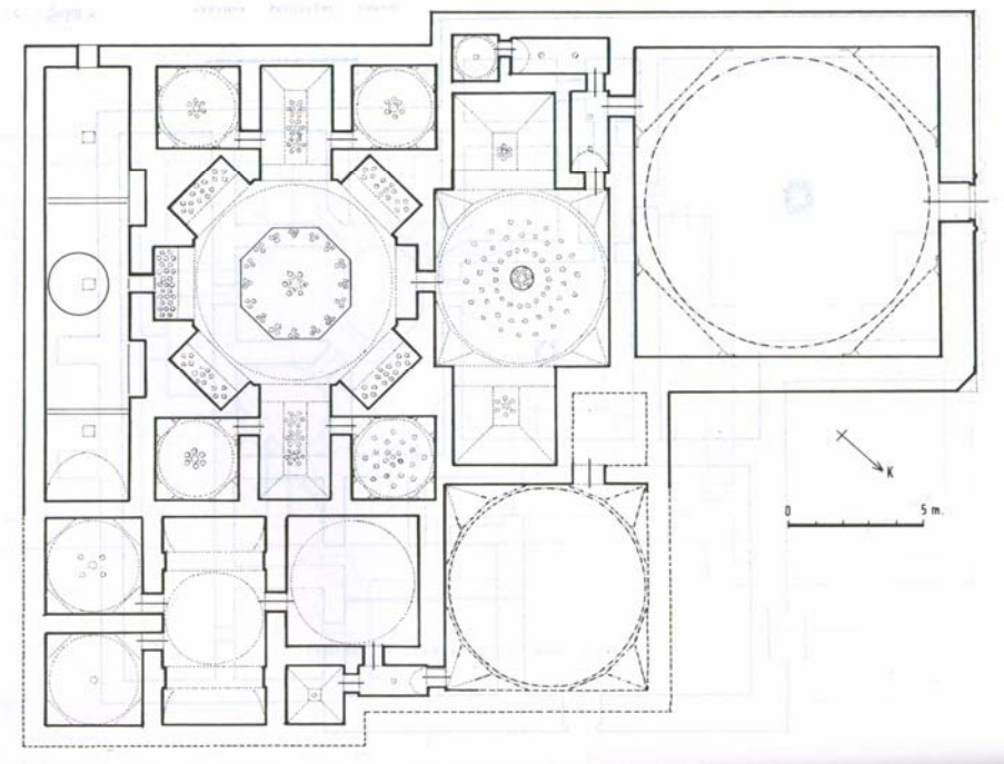
Krş. Planı 5.33: Karaman Yeni Hamamı (Y. Önge'den)
