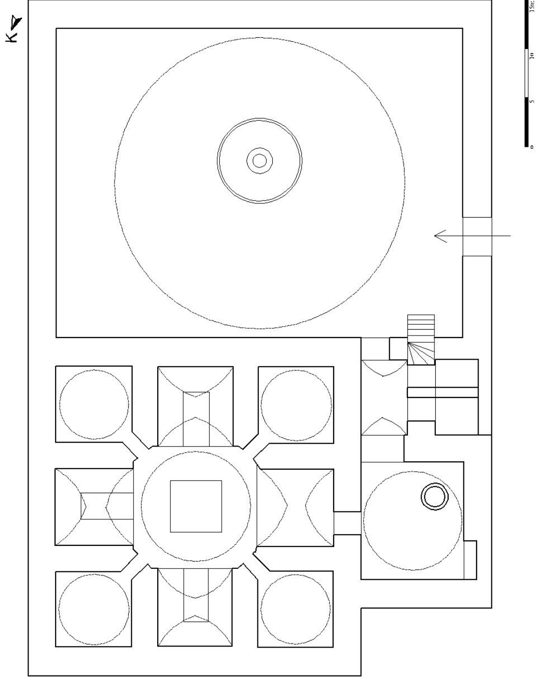
Plan 4.7: Erzurum Kırkçeşme Hamamı (R.H.Ünal'dan düzeltilerek)
