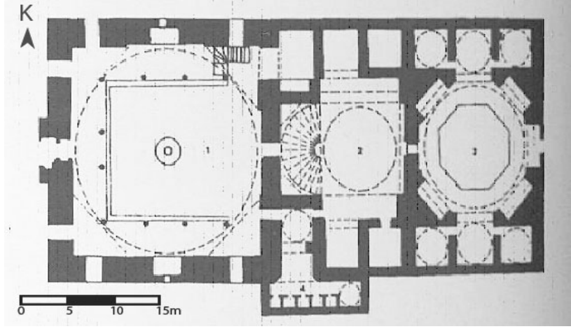
Krş. Planı 5.23: İstanbul Mahmut Paşa Hamamı (O. Aslanapa'dan)
