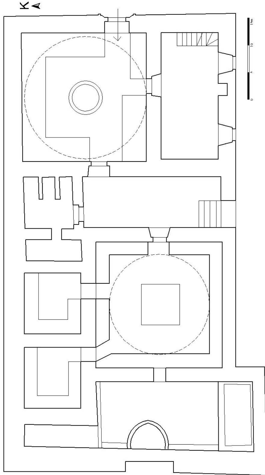
Plan 4.9: Erzurum Askeri Hamam (V.G.M.'den)
