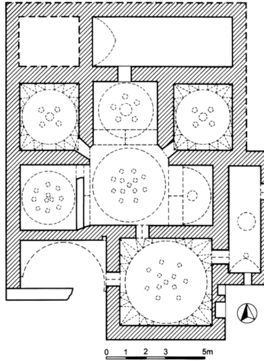
Krş. Planı 5.22: Afyon Zile Işıklı Hamamı ( www.ayfon.bel.tr )
