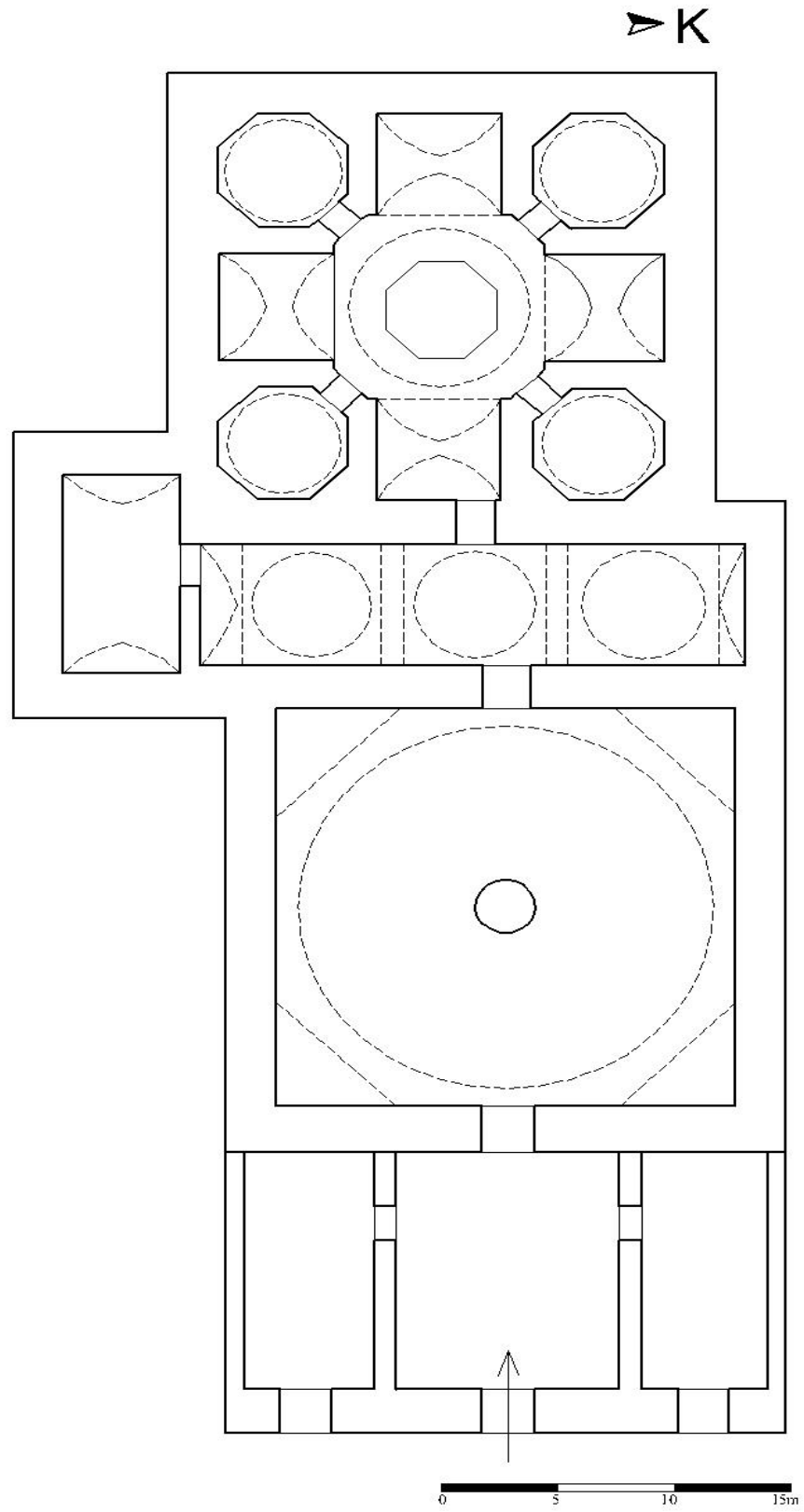
Plan 4.17: Erzurum Şeyhler Hamamı (R. H. Ünal'dan düzeltilerek)
