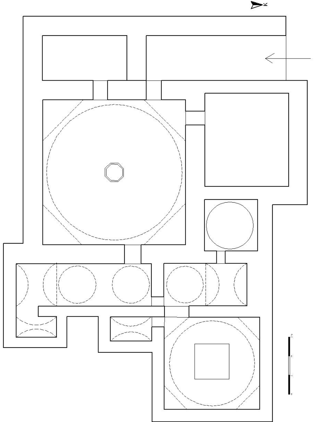
Plan 4.8: Erzurum Küçük Hamam (V.G.M.'den)
