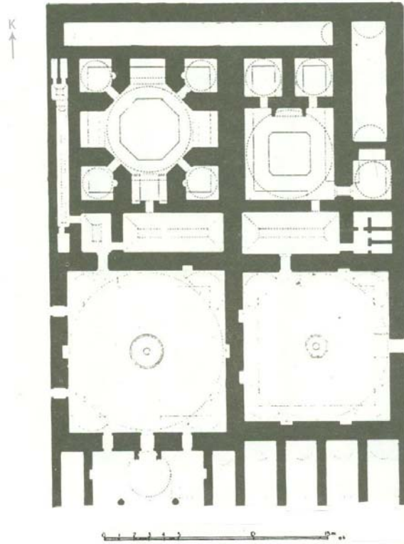
Krş. Planı 5.10: Edirne Sokullu Mehmet Paşa Hamamı (Y. Önge'den)
