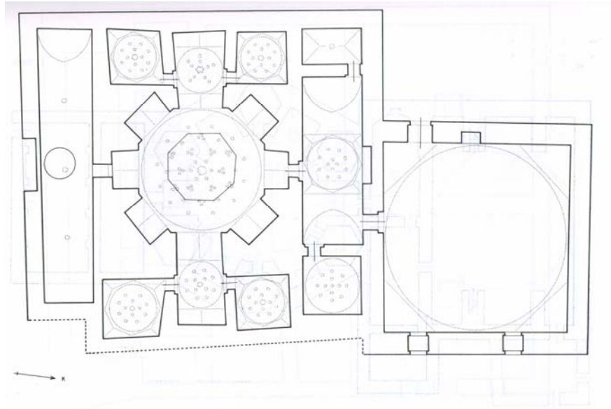
Krş. Planı 5.24: Konya Ereğli Eski Hamamı (Y. Önge'den)
