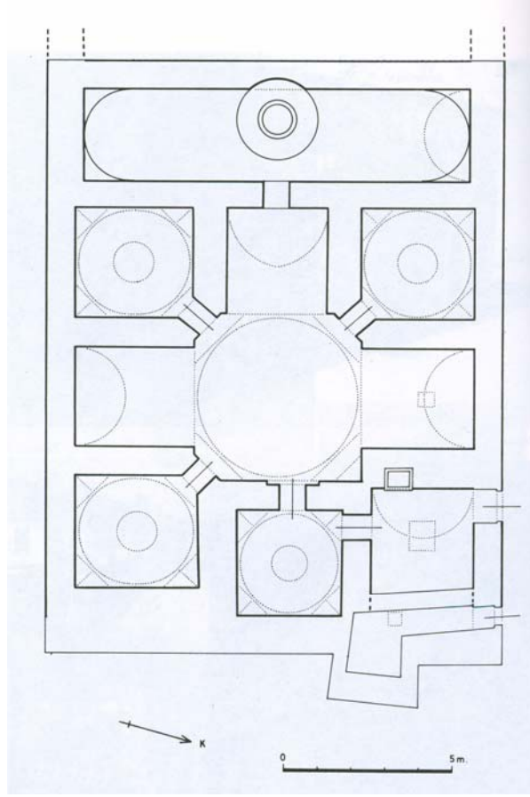
Krş. Planı 5.17: Kastamonu Frenkşah Hamamı (Y. Önge'den)
