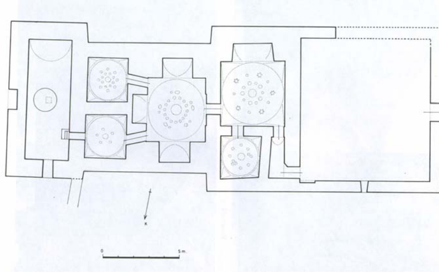
Krş. Planı 5.21: İçel Mamuriye Hamamı (Y. Önge'den)
