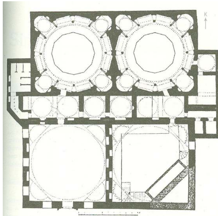
Krş. Planı 5.26: Çemberlitaş Nurbanu Valide Sultan Hamamı (Y. Önge'den)
