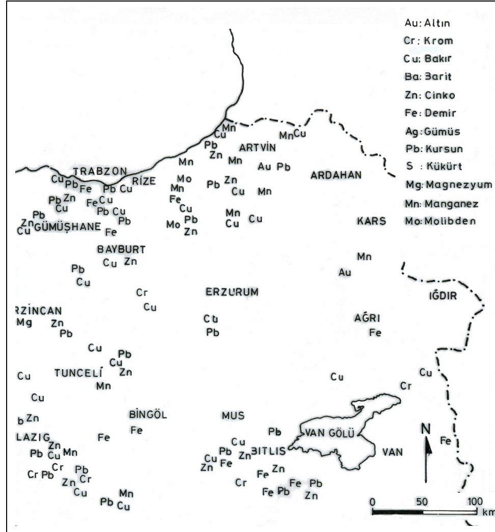
Harita 2: Doğu Anadolu ve Doğu Karadeniz Bölgeleri Maden Kaynakları.
