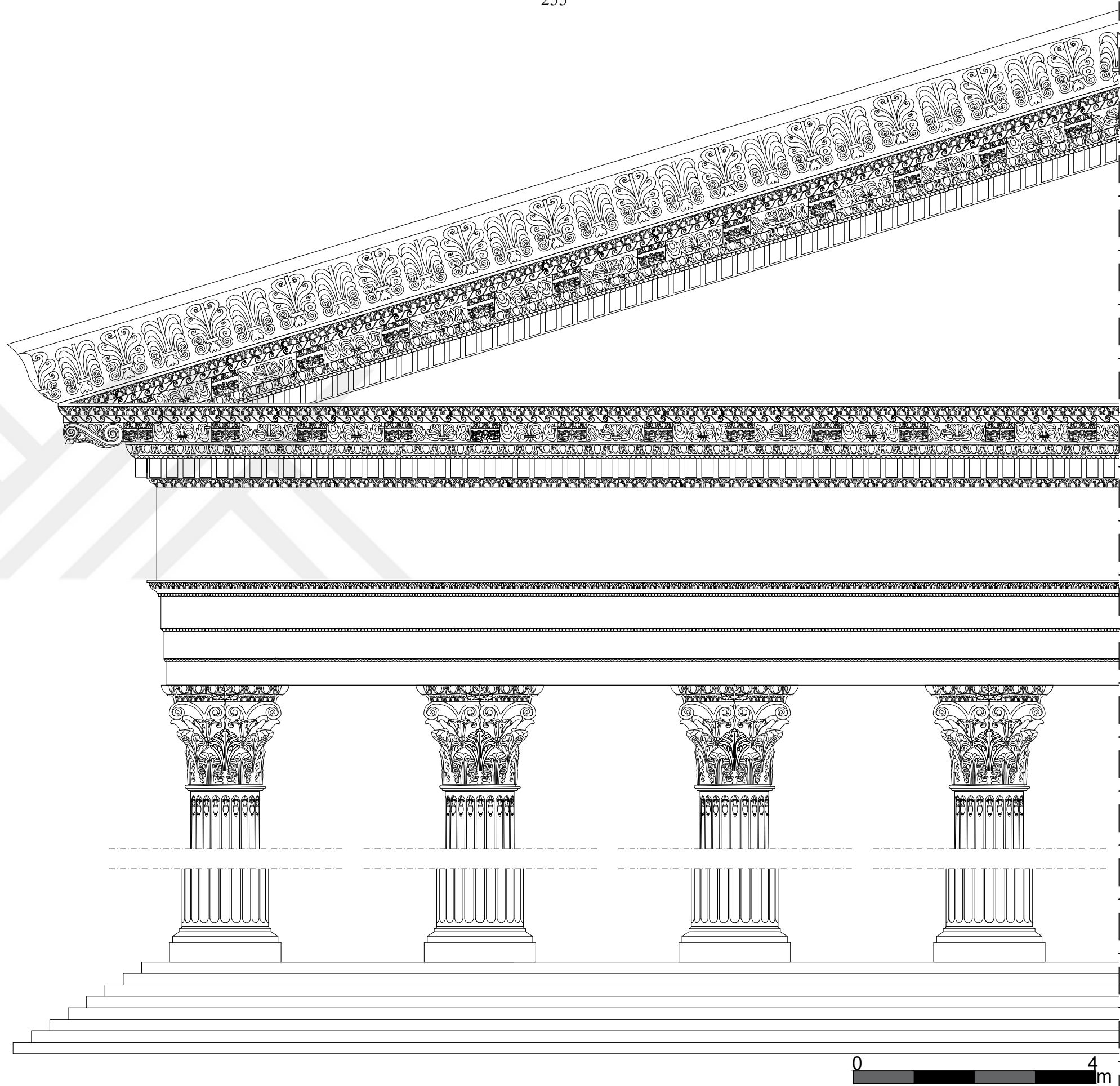
Çizim 8. Tapınak Doğu Kısa Kenar Yeniden Kurma Denemesi
