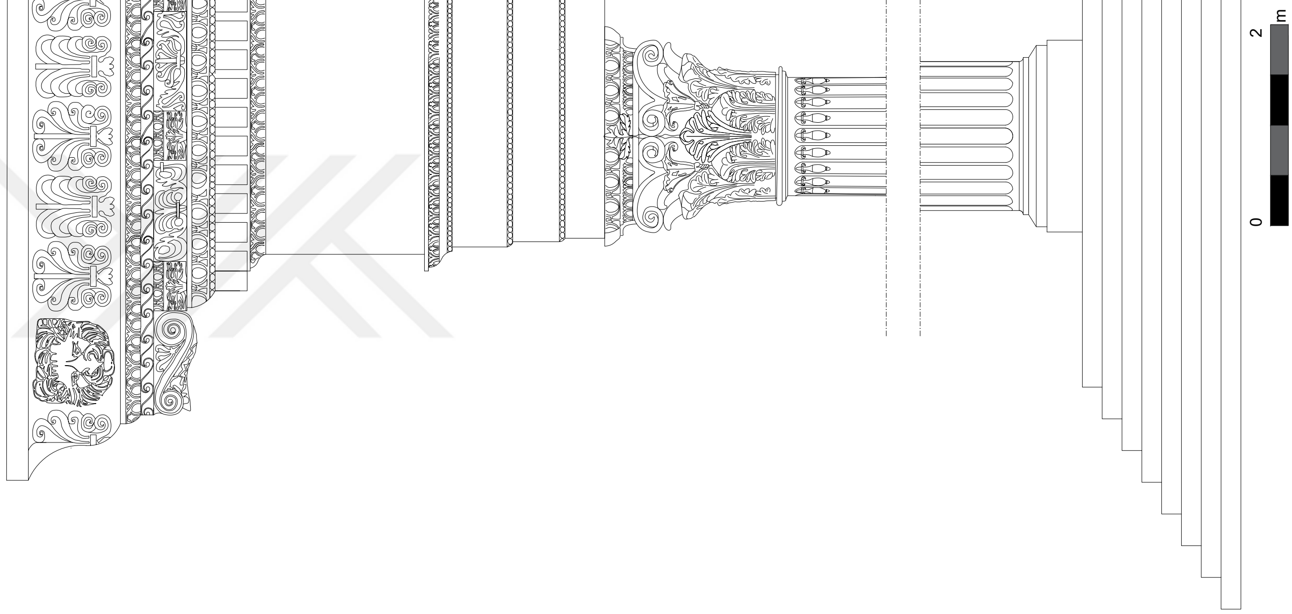
Çizim 4. Tapınak Güney Uzun Kenar Yeniden Kurma Denemesi
