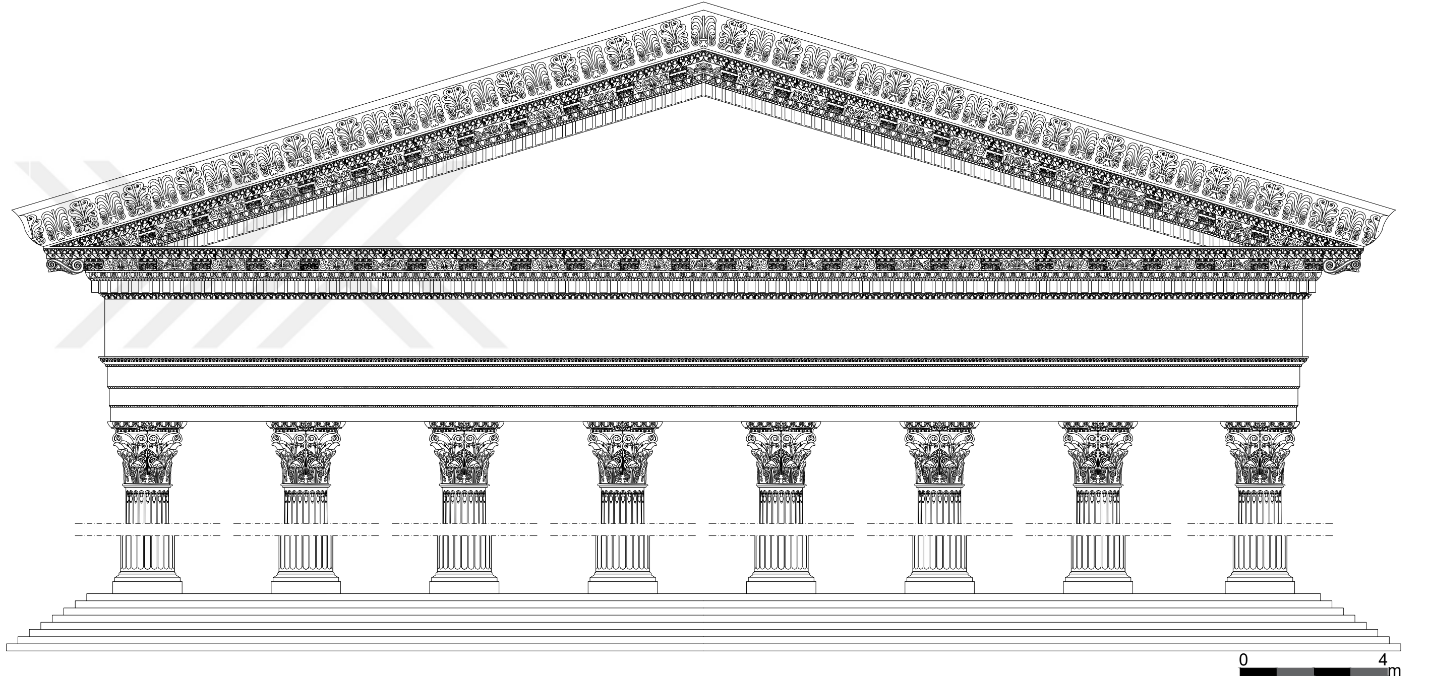
Çizim 7. Tapınak Doğu Kısa Kenar Yeniden Kurma Denemesi
