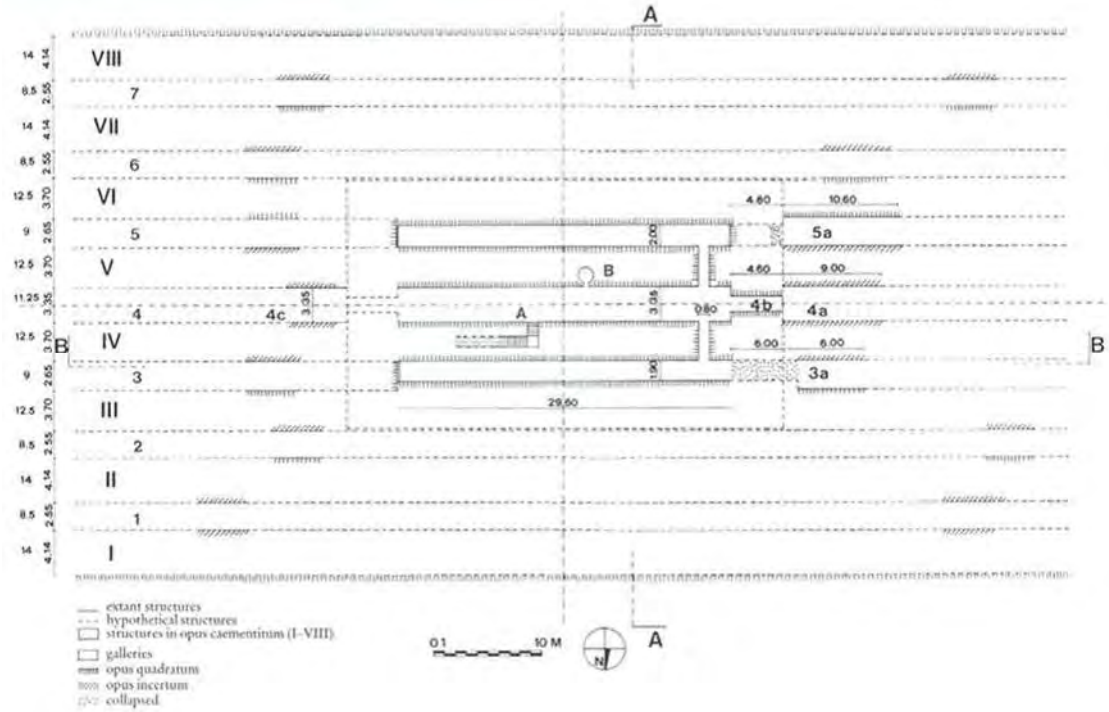
Çizim 2. Kyzikos Hadrian Tapınağı Alt Yapı Planı (Weißmann, 2013, Tafel 19.2)
