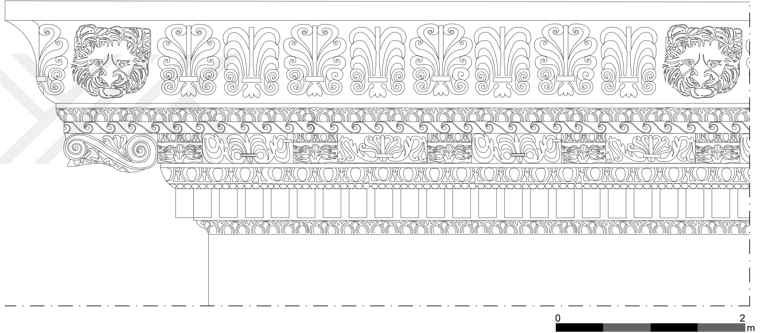
Çizim 5. Tapınak Güney Uzun Kenar Yeniden Kurma Denemesi
