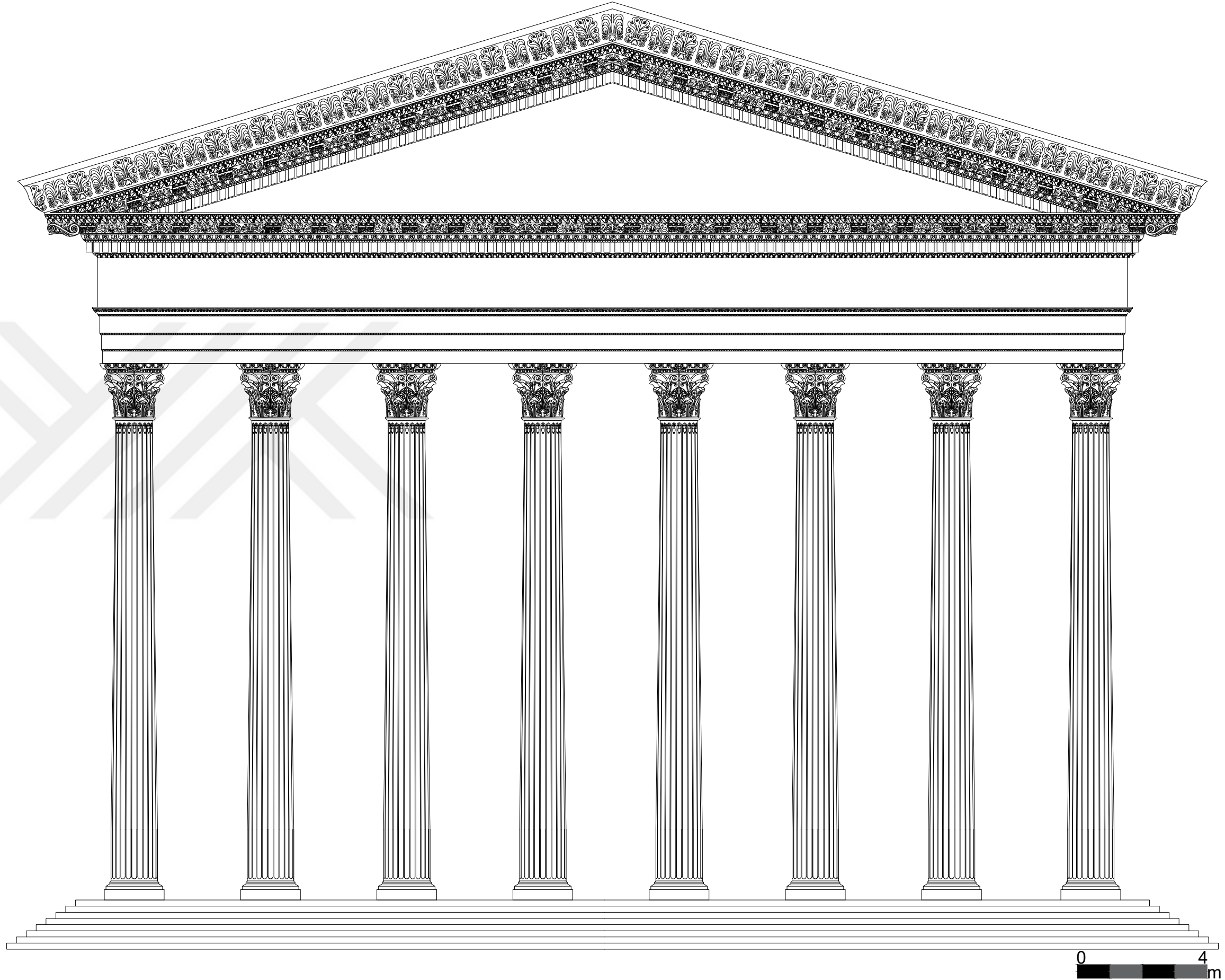
Çizim 6. Tapınak Doğu Kısa Kenar Yeniden Kurma Denemesi
