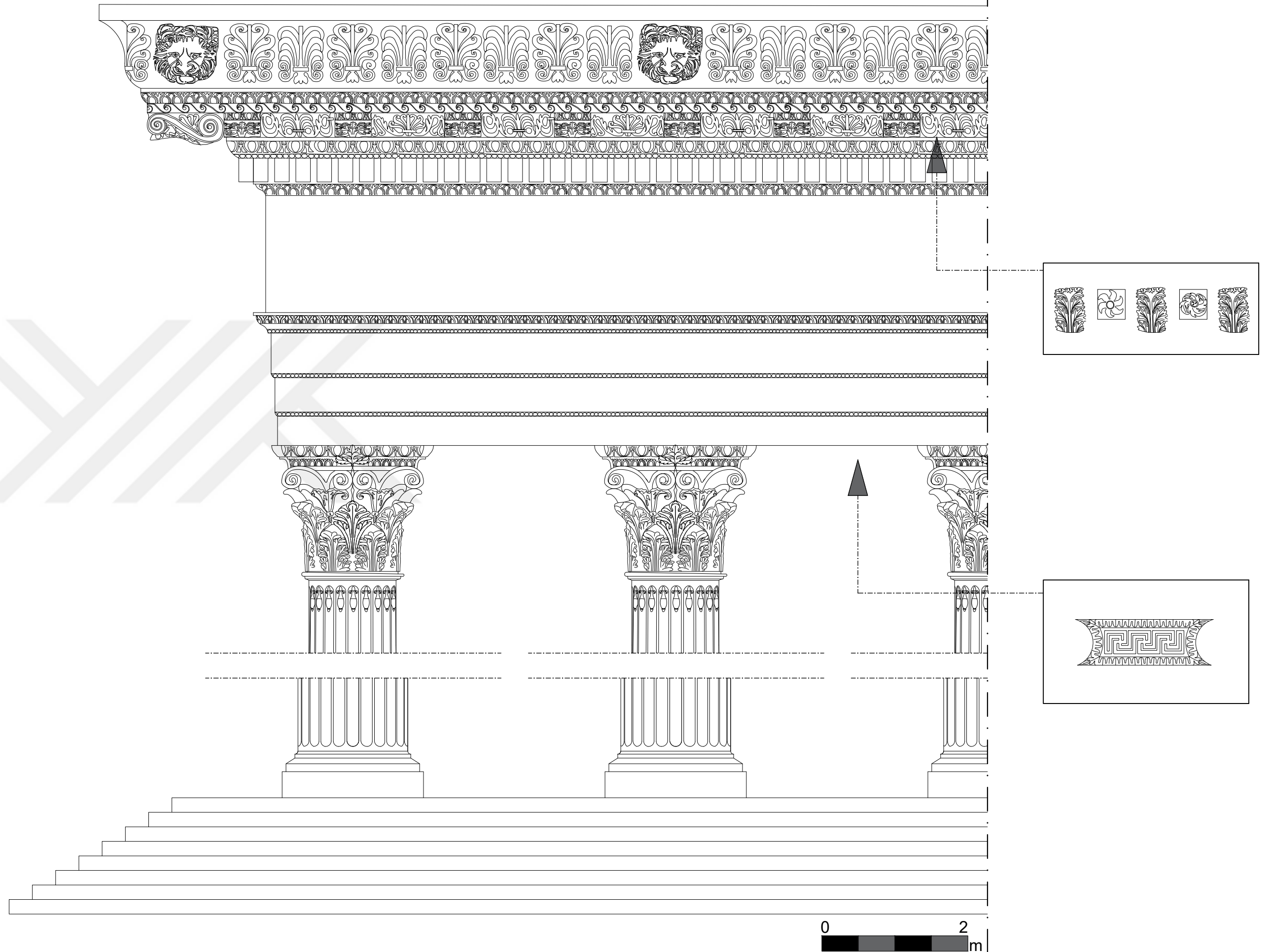
Çizim 3. Tapınak Güney Uzun Kenar Yeniden Kurma Denemesi
