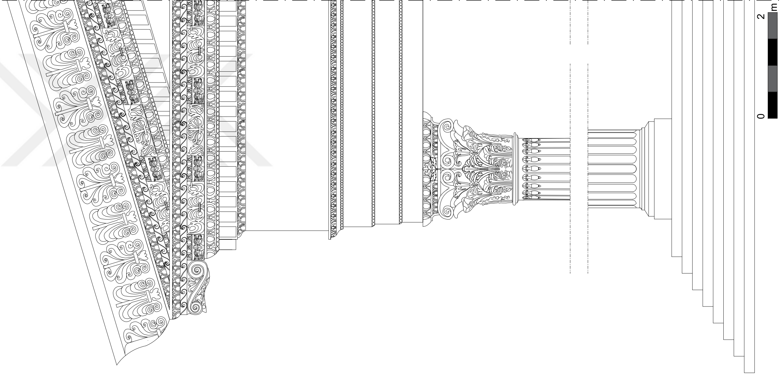
Çizim 9. Tapınak Doğu Kısa Kenar Yeniden Kurma Denemesi
