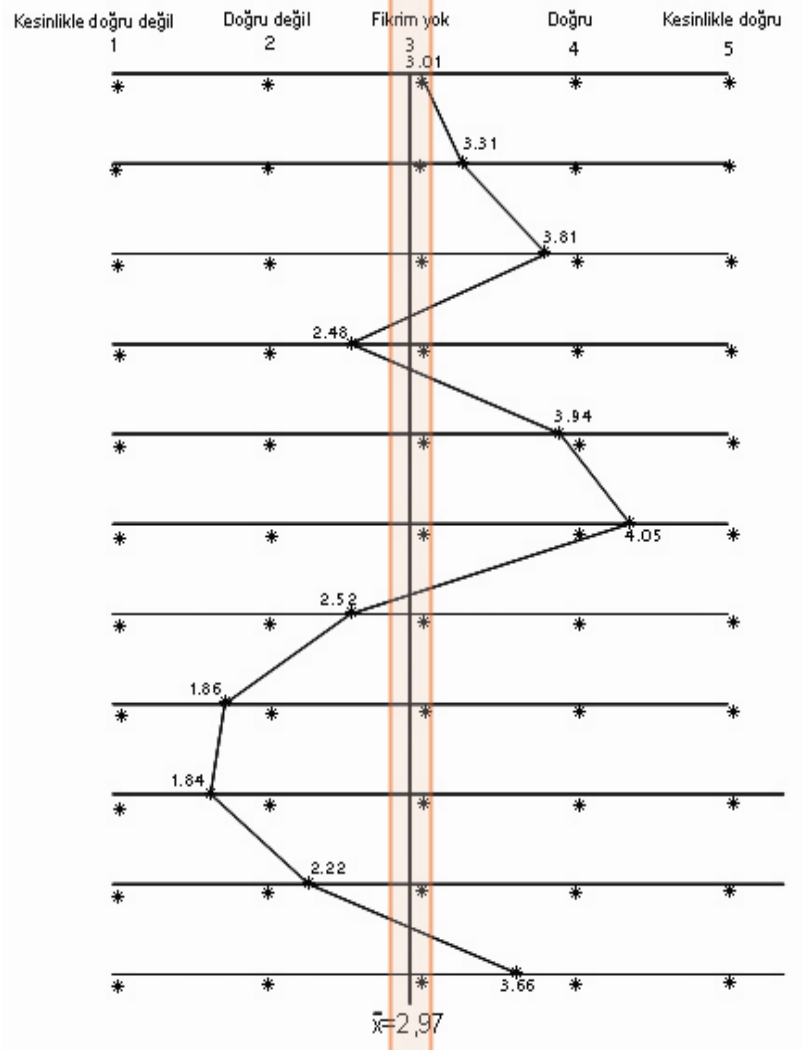
Şekil 4.21: Göç Nedenlerinin Ortalama Değerleri için Önemlilik ve Karasızlık Bandı
