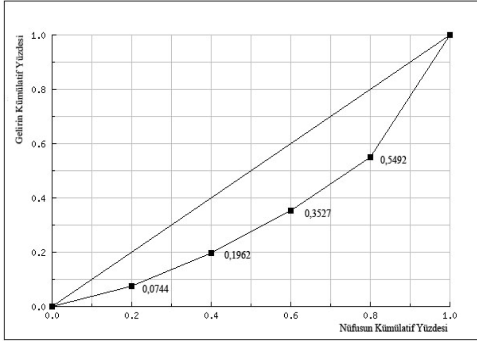
Şekil 4.22: Ağrı İlinde %20'lik Gruplara Göre Lorenz Eğrisi
