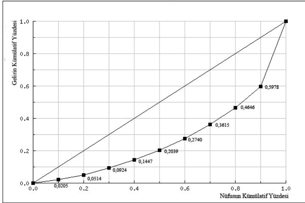
Şekil 4.32: Kars İlinde %10'luk Gruplara Göre Lorenz Eğrisi
