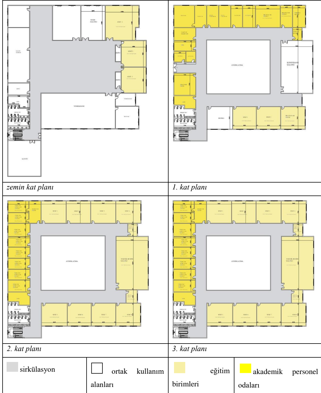
Çizelge 4.8. P4 kodlu yapı kat planları
