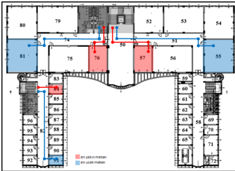
Şekil 5.11. Ortak mekanlar
