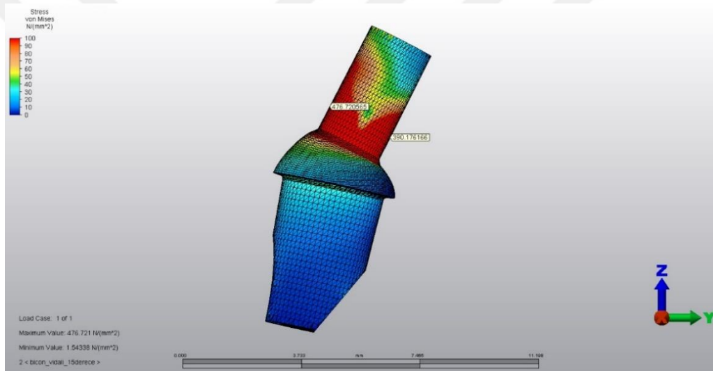
Şekil 4.17. Kısa Vidalı 15° Abutmentteki von Mises Stresleri
