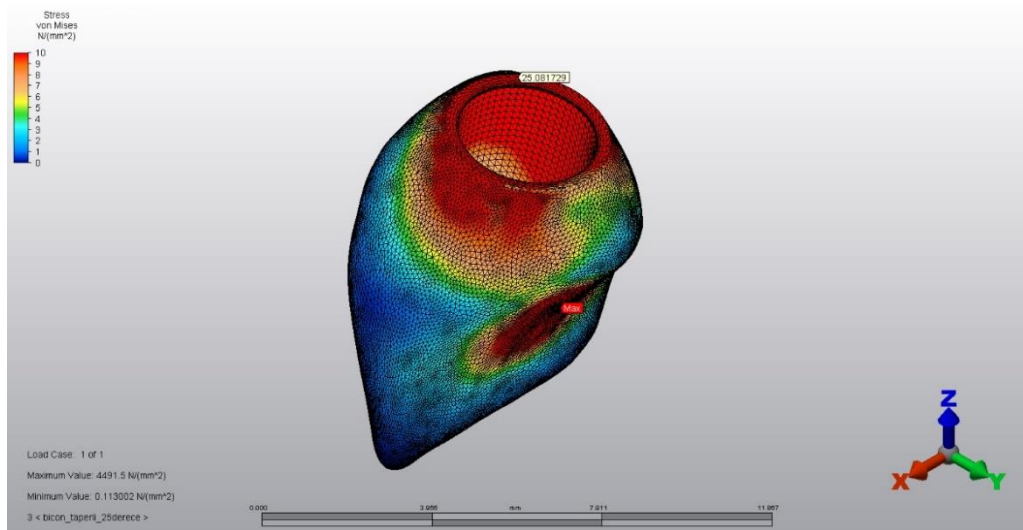
Şekil 4.21. Kısa Taper 25° Kuronundaki von Mises Stresleri
