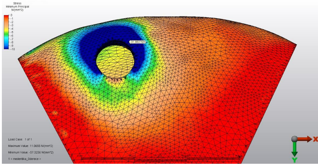
Şekil 4.31. Normal 0° Kortikal Kemik Üzerindeki Basma Stres Değerleri
