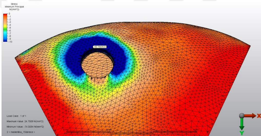
Şekil 4.32. Normal 15° Kortikal Kemik Üzerindeki Basma Stres Değerleri
