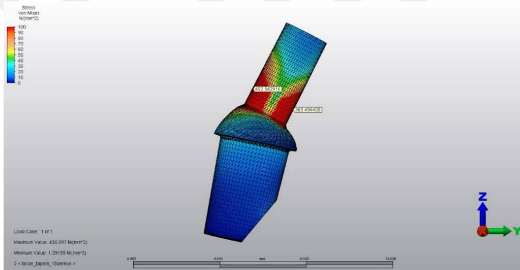
Şekil 4.11. Kısa Taper 15° Abutmentteki von Mises Stresleri
