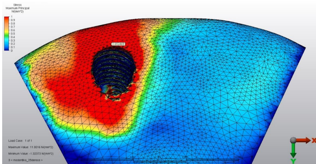
Şekil 4.60. Normal 25° Kansellöz Kemik Üzerindeki Çekme Stres Değerleri
