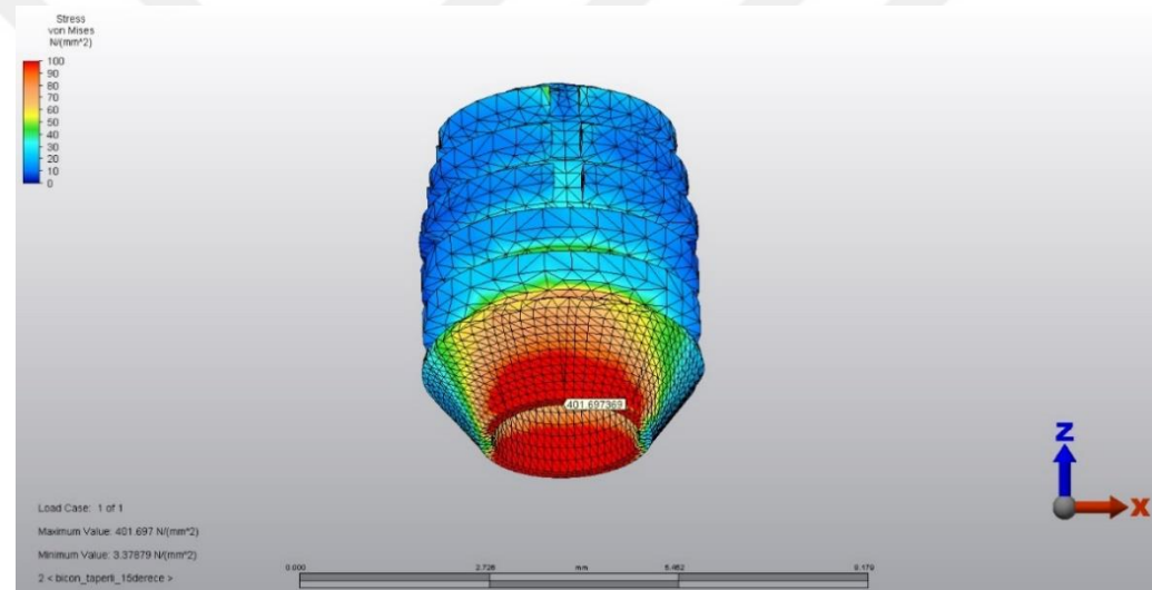
Şekil 4.2. Kısa Taper 15° İmplanttaki von Mises Stresleri
