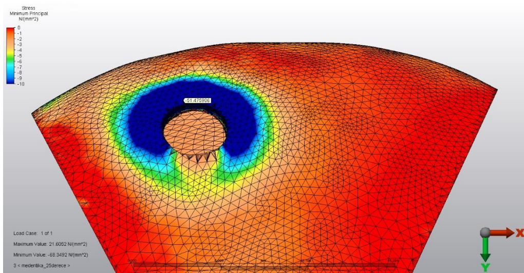
Şekil 4.33. Normal 25° Kortikal Kemik Üzerindeki Basma Stres Değerleri
