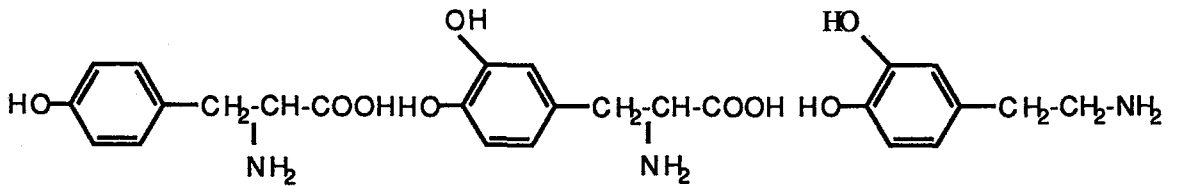
(XV) Tirozin
