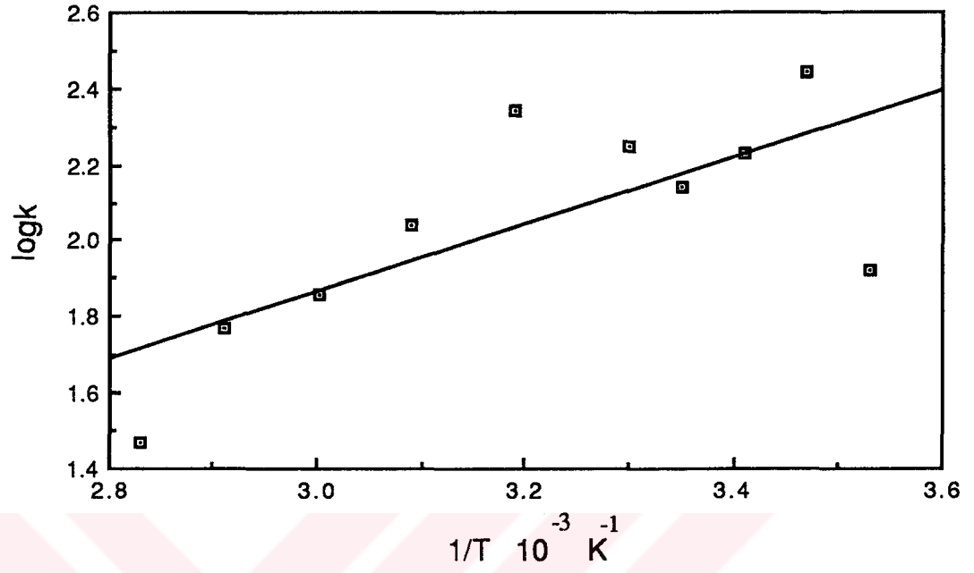
Şekil 3.27. Kuşburnu meyvası PPO enzimi için pirogallol substratı ile elde edilen \log k-(1/T) grafiği
