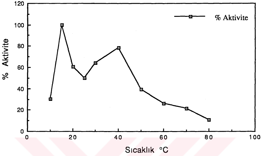
Şekil 3.18. Kuşburnu meyvası PPO enzimi için, 10 mM pirogallo! substratıyla elde edilen sıcaklık - % aktivite grafiği
