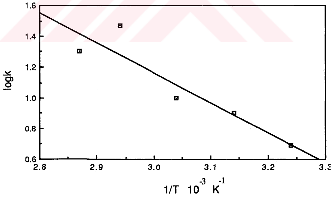
Şekil 3.28. Kuşburnu meyvası PPO enzimi için L-tirozin substratı ile elde edilen \log k-(1/T) grafiği
