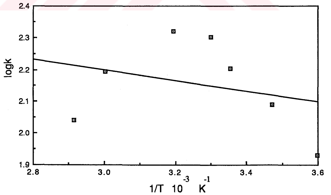
Şekil 3.26. Kuşburnu meyvası PPO enzimi için gallik asit substratı ile elde edilen \log k - (1/T) grafiği
