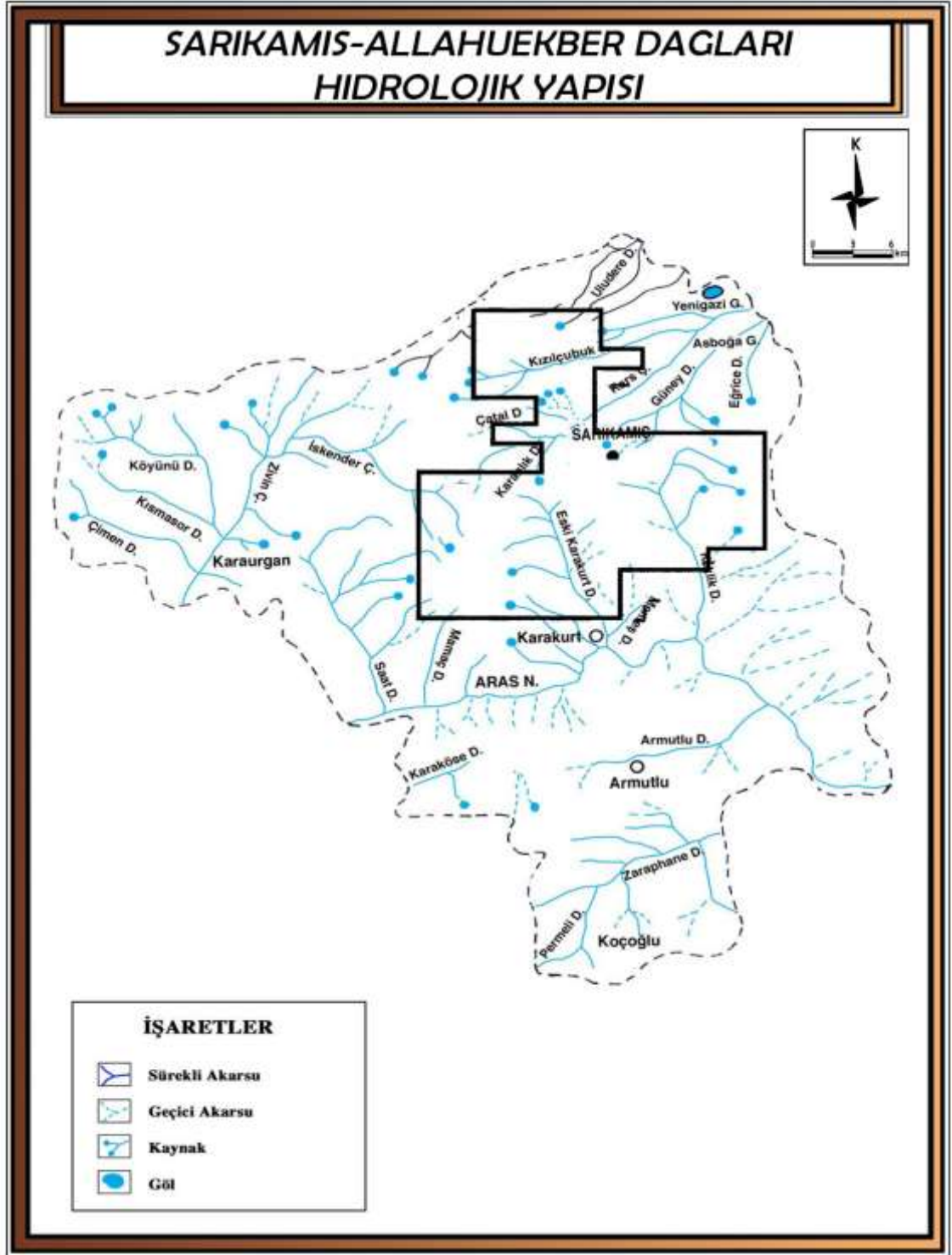
Şekil 5. Sarıkamış-Allahuekber Dağları hidrolojik yapısı (Özer, 2004)
