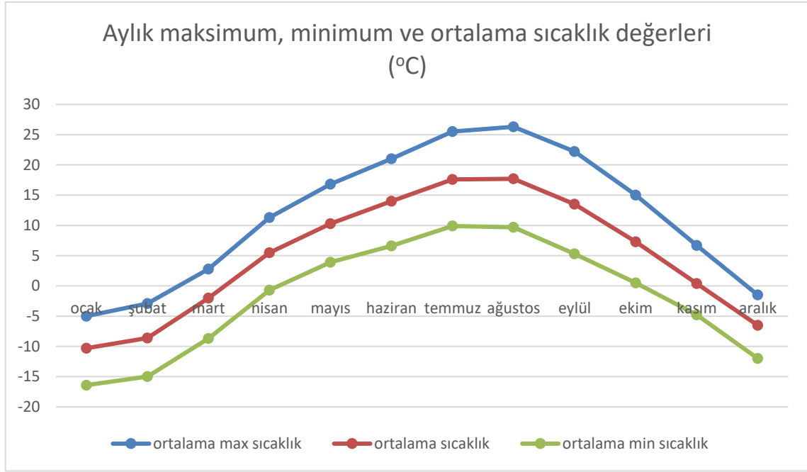
Şekil 4. Sarıkamış aylık maksimum, minimum ve ortalama sıcaklık değerleri (°C) grafiği
