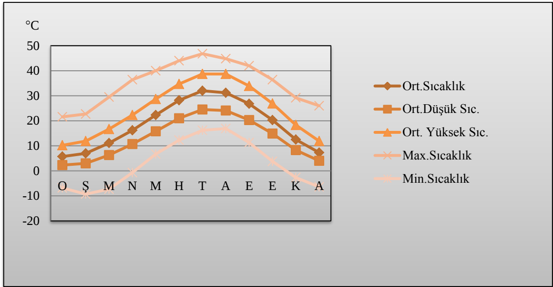
Şekil 2.1. Şanlıurfa'nın Sıcaklık Değerlerinin Yıl İçindeki Seyri (1970-2013).
