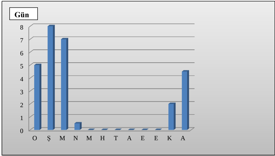
Şekil 2.2. Şanlıurfa’da Aylara Göre Donlu Gün Sayısı (1970-2013).
