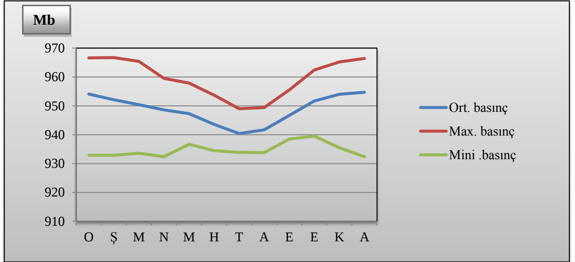
Şekil 2.5. Şanlıurfa'nın Ortalama ve Ekstrem Basınç Değerlerinin Aylara Göre Dağılımı (1970-2013).
